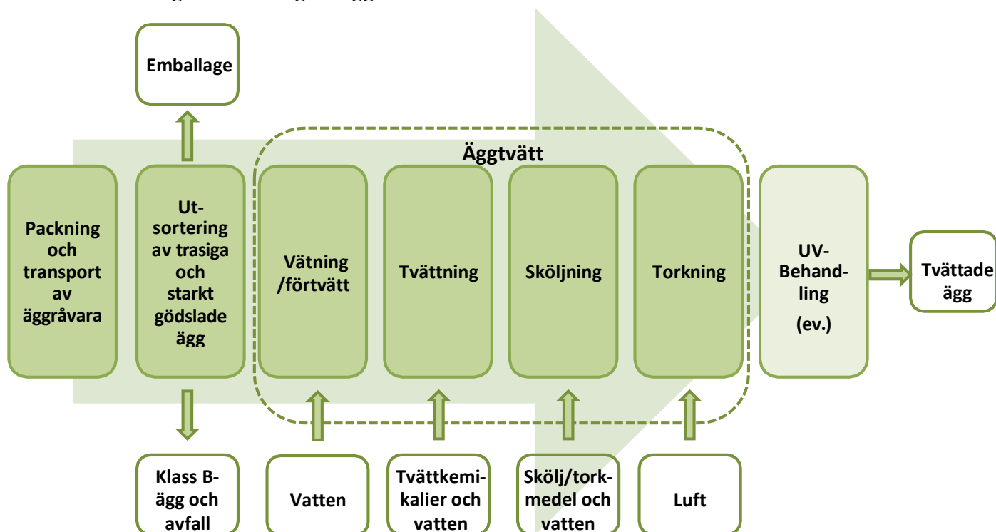
Figur 3. Principskiss över de olika processtegen vid industriell tvättning av ägg.
